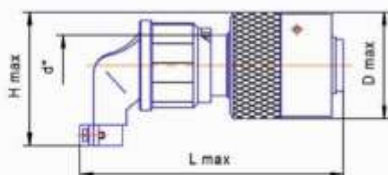
Розетка кабельная с угловым кожухом
