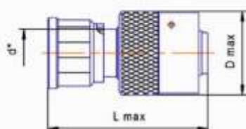
Розетка кабельная
