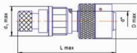
Розетка кабельная с обложкой под термоусаживающиеся трубки
